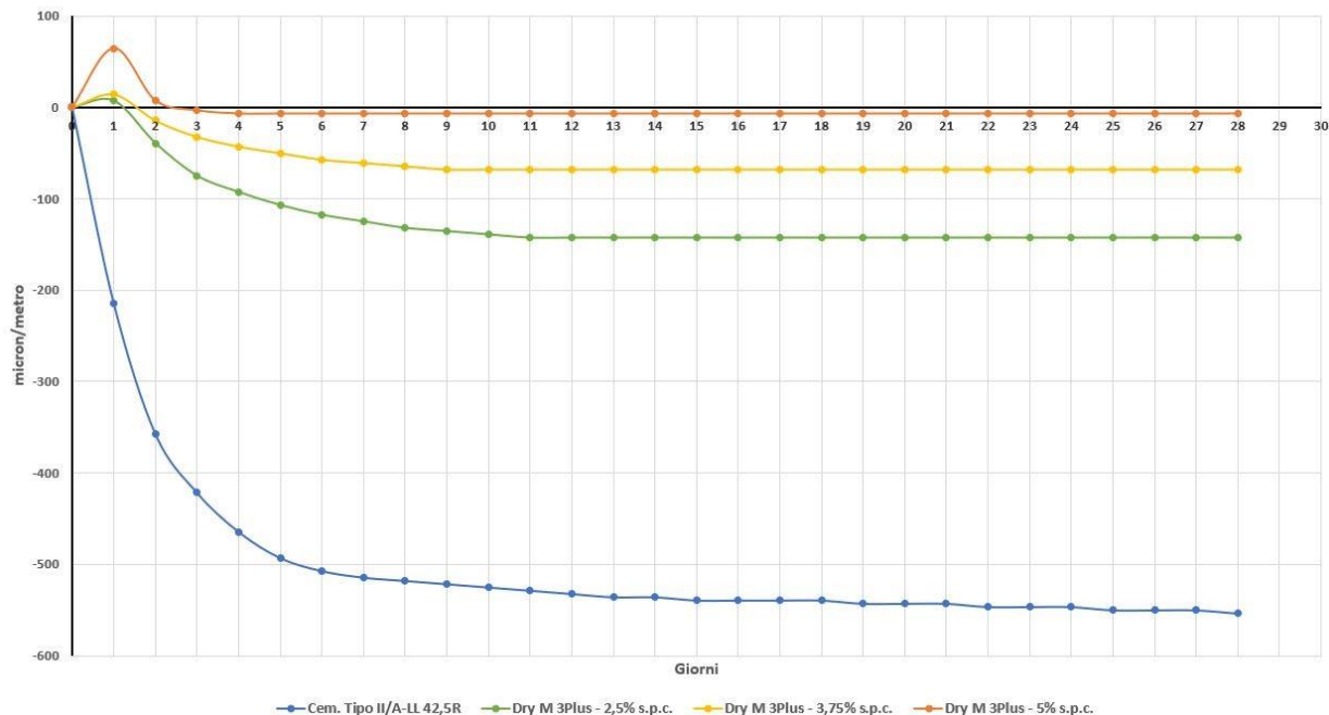
DRY M 3Plus - Espansione/Ritiro Libero su Malta (met. UNI 8147 mod.)
